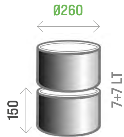
VETRINA A 2 FILE CON CARAPINE DA Ø26 CM 2-ROW DISPLAY CASE WITH PANS OF Ø26 CM
